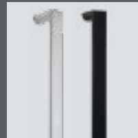
Griffstange mit geraden Stützen und gerundeter Rückseite, Edelstahl in vier Längen (800, 1.200, 1.400, 1.600 mm). Auch in Schwarz (gegen Mehrpreis). Auch mit Fingerscan bei den Längen 1.200 und 1.600 mm.
